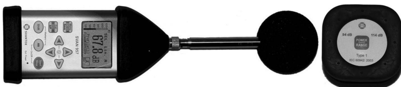
51 pav. SVAN 957 Triukšmo ir vibracijos matuoklis.
