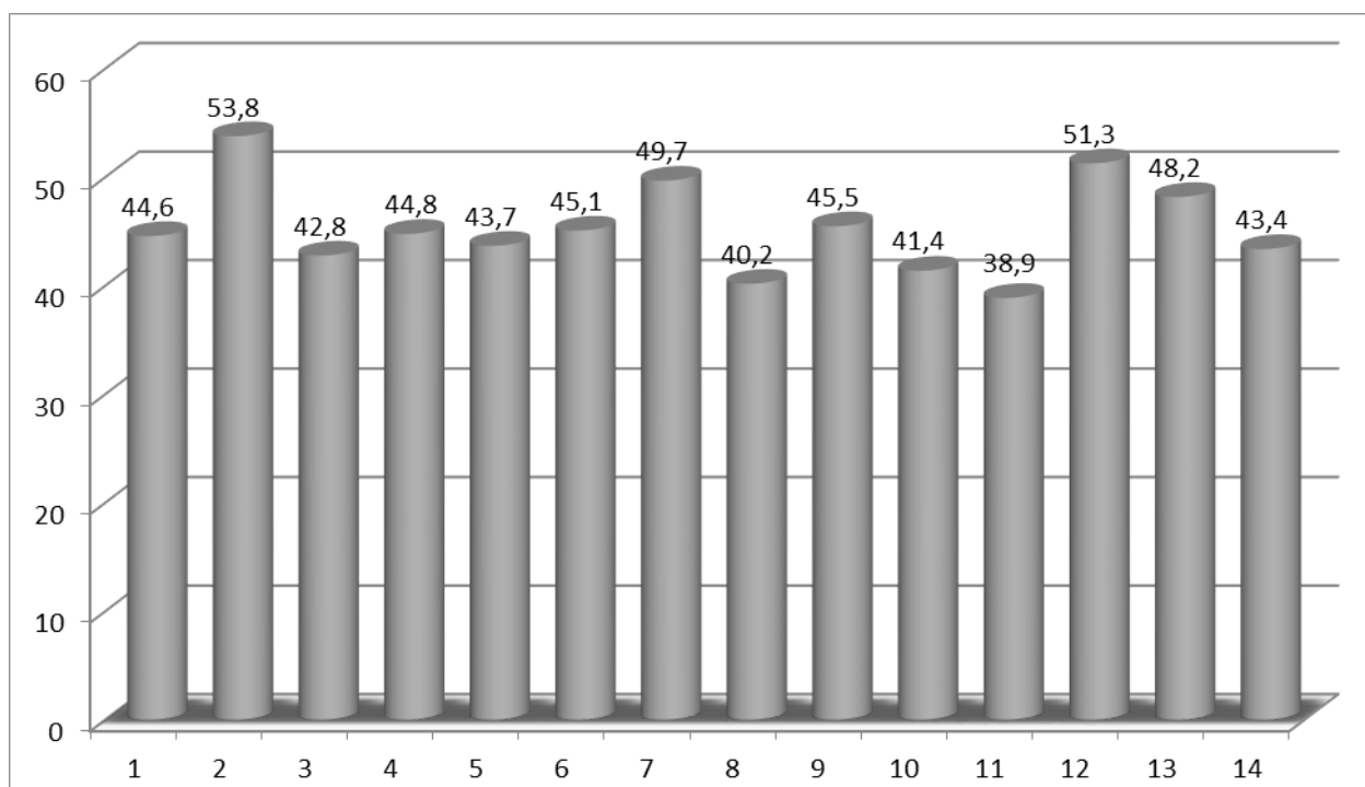
65 pav. Ekvivalentinio triukšmo pasiskirstymas matavimo vietose nakties metu (22-7 val.). Ribinis dydis 55 dBA.
