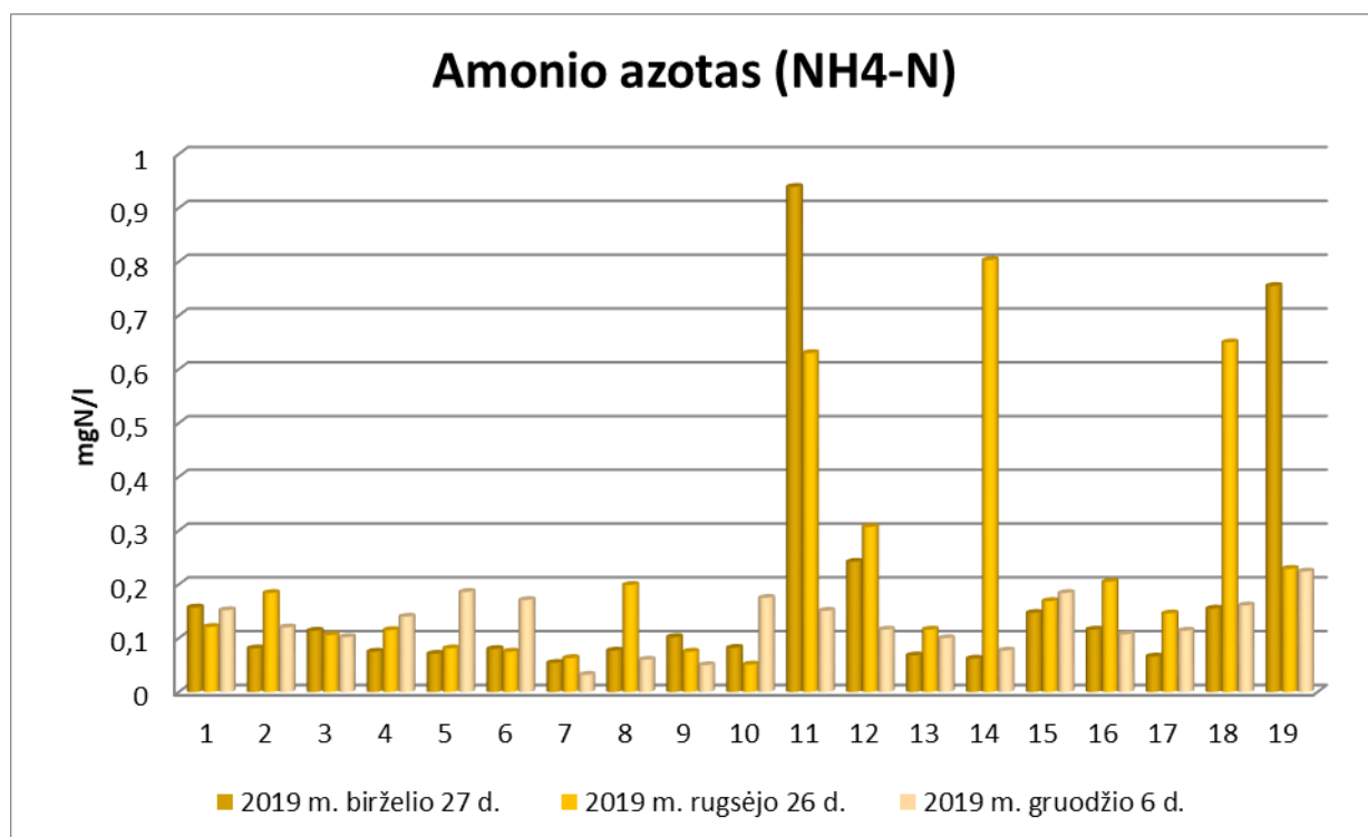
24 pav. Amonio azoto koncentracijos kitimas per 2019 m.
