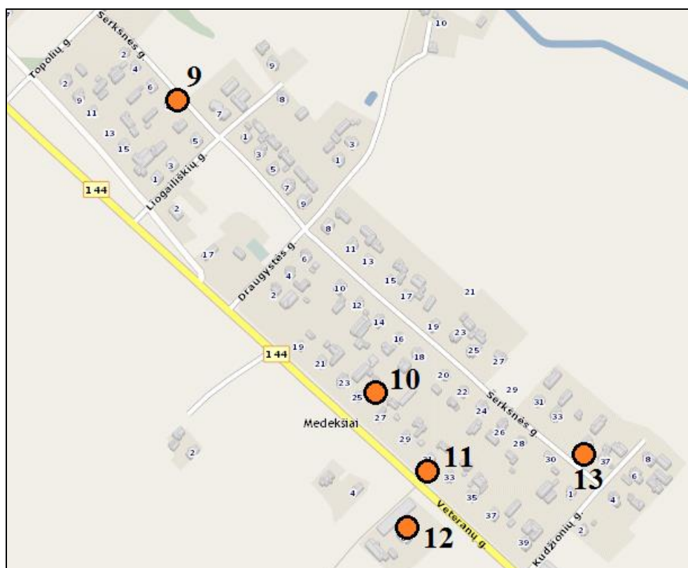
38 pav. Požeminio vandens monitoringo tinklas Medėkšių gyv., Palėdnagių sen.
